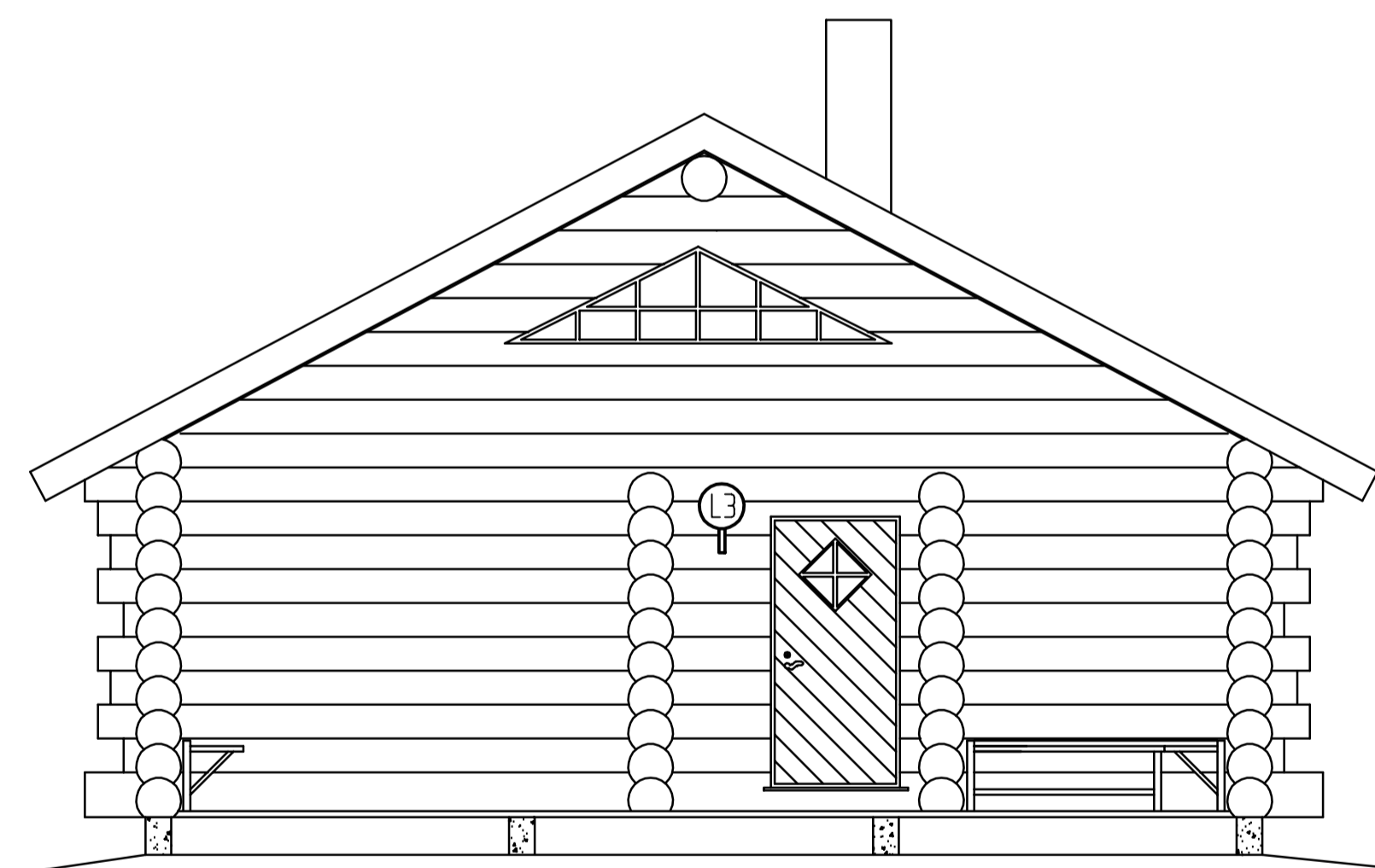
JULKISIVU, POHJOINEN
