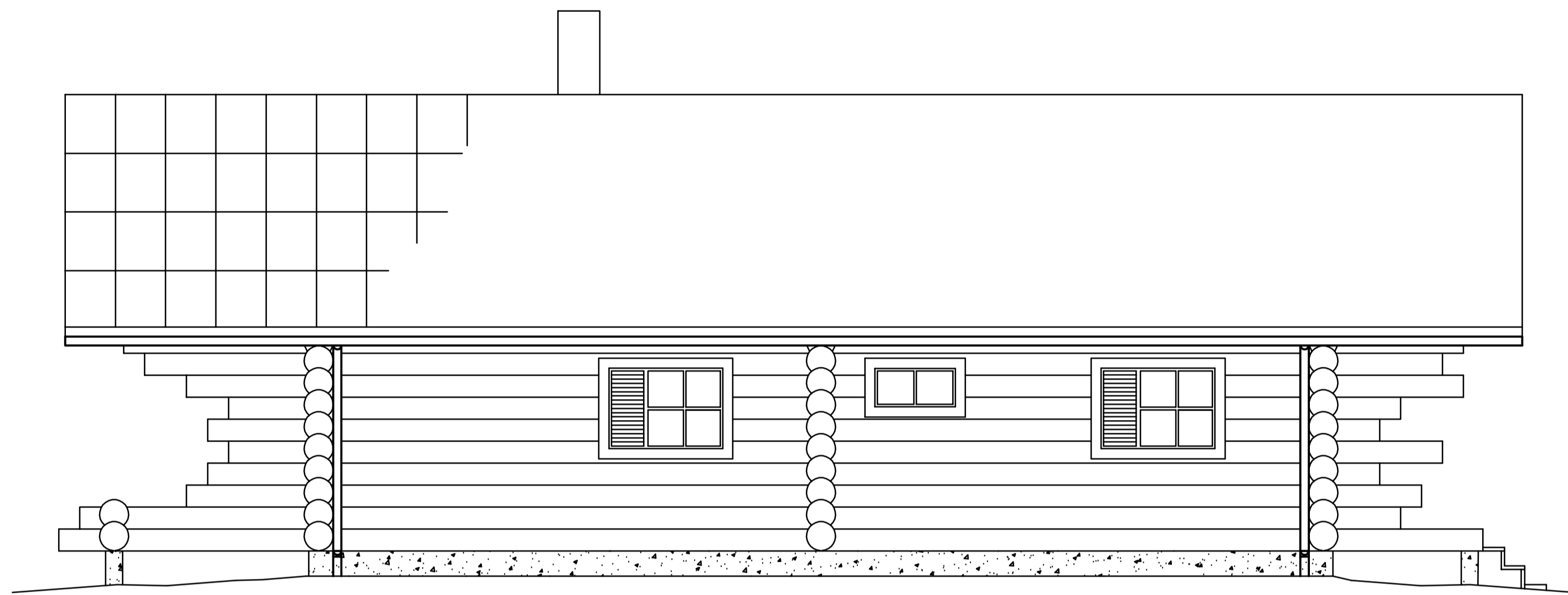
JULKISIVU, ITÄ
