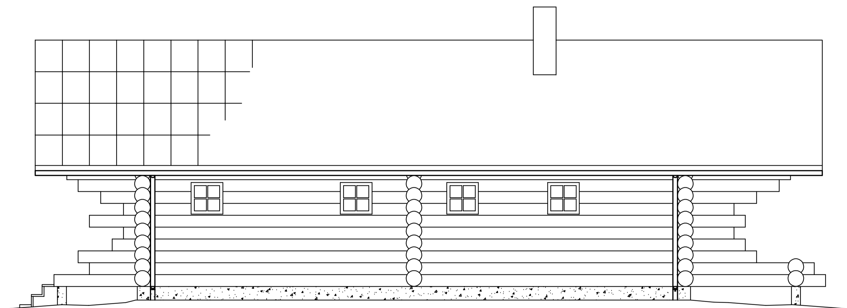
JULKISIVU, LÄNSI
